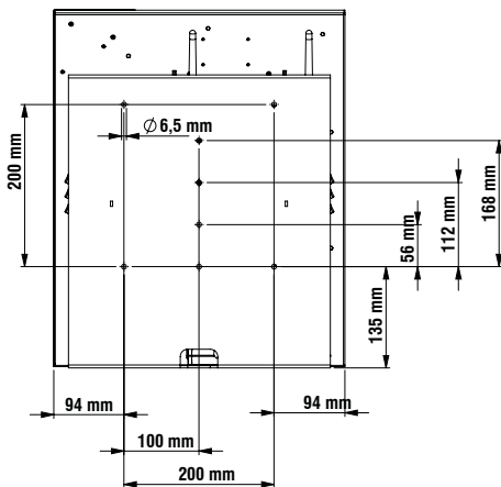
Variant Flex 21.5 lite inkl. Zebra Scanner und Zahlungsmodul
