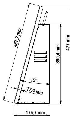
Variant Flex 21.5 lite inkl. Zebra Scanner und Zahlungsmodul
