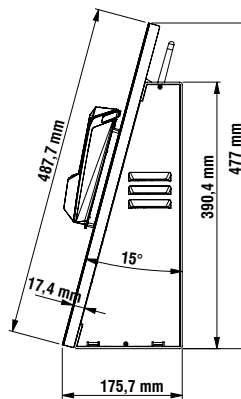
Variant Flex 21.5 lite inkl. Magellan Scanner, Zahlungsmodul und beleuchtetem Acryl auf der Oberseite
