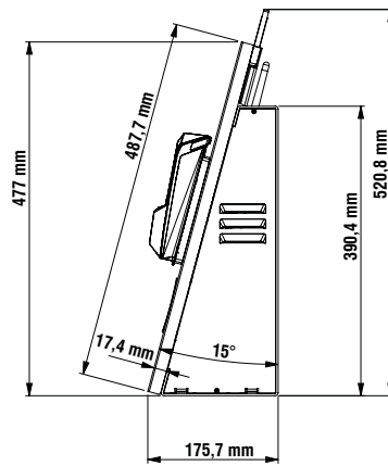
Variant Flex 21.5 lite inkl. Magellan Scanner, Zahlungsmodul und beleuchtetem Acryl auf der Oberseite
